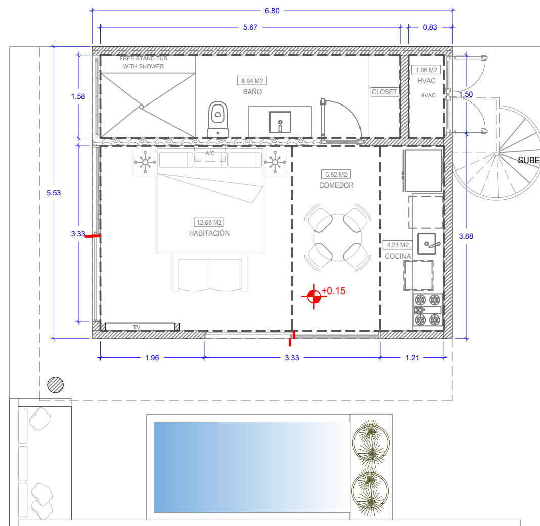
PLANTA TIPO VILLA (A) - 37.05 M2 ESPESOR MUROS 15CM - (4.32 M2) ÁREA EXTERIOR - (23.72 M2) ÁREA DEL TERRENO - (91.47 M2)
