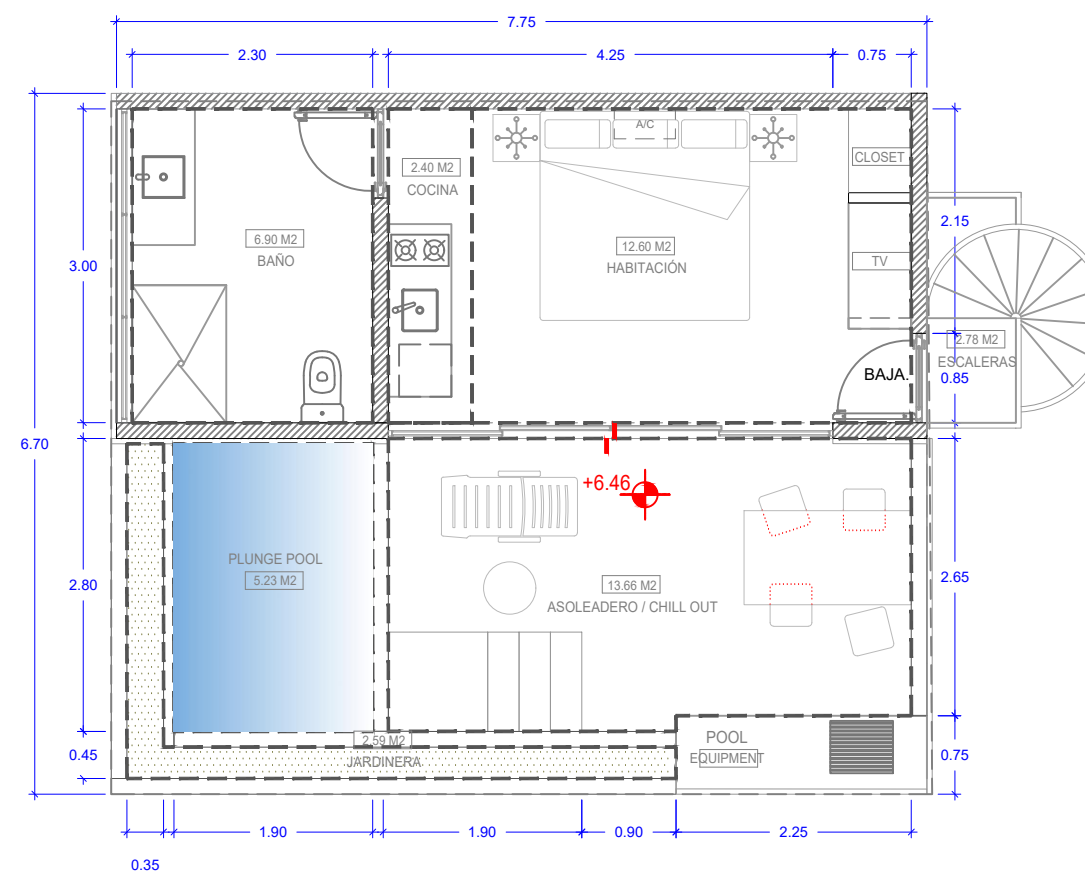
PLANTA TIPO VILLA (A) - 54.63 M2 ESPESOR MUROS 15CM - (10.87 M2)
